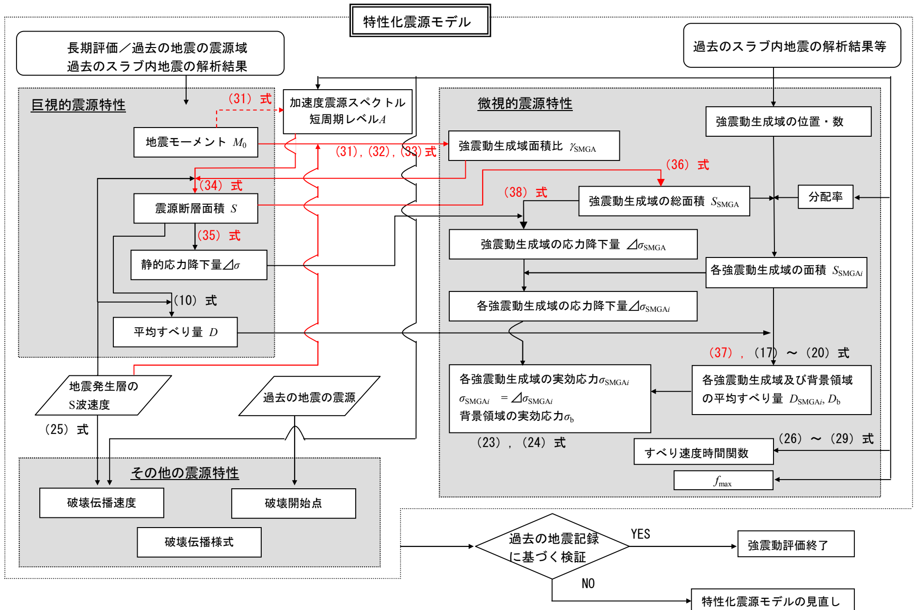
付図6 スラブ内地震の震源特性パラメータ設定の流れ (赤がプレート境界地震の流れからの変更点)
